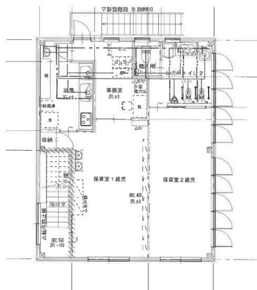
2階平面図 S=1:100
