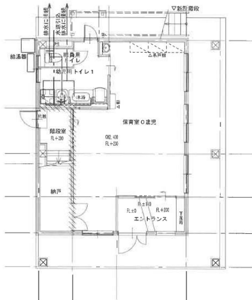
1階平面図 S=1:100
